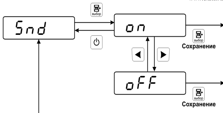
Рисунок 5.4 Включение / выключение звуковой сигнализации нарушения порога
