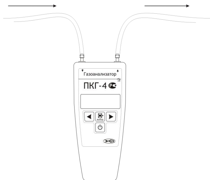
Рисунок 5.7 Схема включения ПКГ-4-СО-К-1 в режиме внешней прокачки газа
