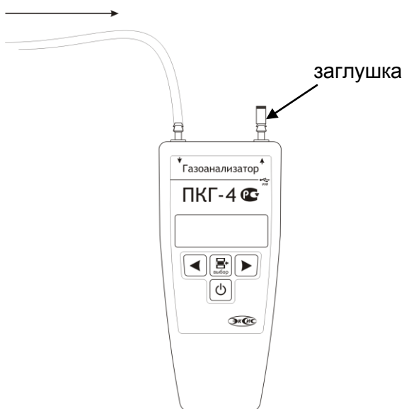
Рисунок 5.6 Схема включения ПКГ-4-СО-К-1 при работе внутреннего побудителя расхода
