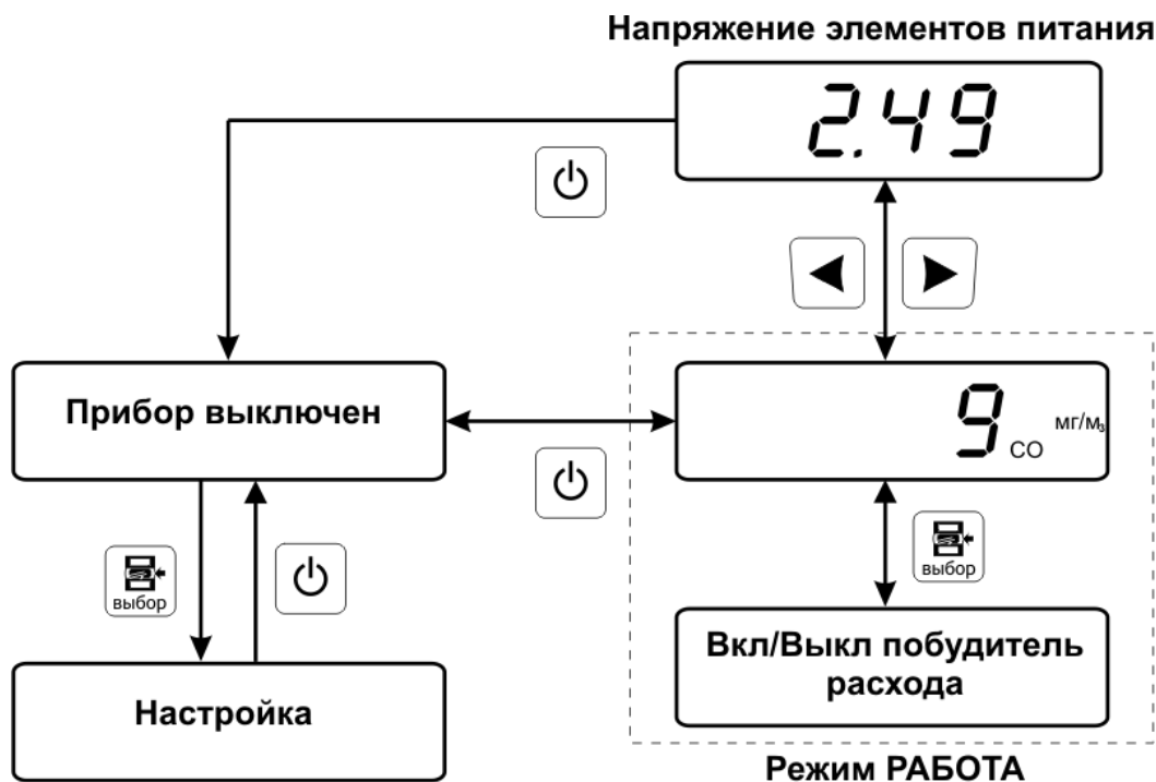
Рисунок 5.1 Схема режима РАБОТА ПКГ-4-СО-К-1
